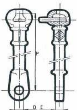
Ball-socket pour travaux sous tension avec carré pour fixation des protections.
