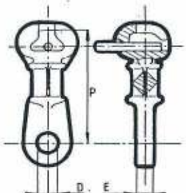
Ball-socket avec carré pour fixation des protections.
