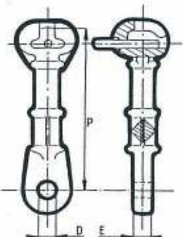
Ball-socket pour isolateur type «Fog» avec carré pour fixation des protections.
